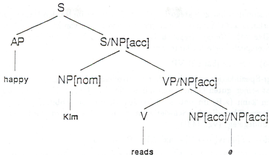
Abbildung 8: Probleme mit der Terminierung von slash
