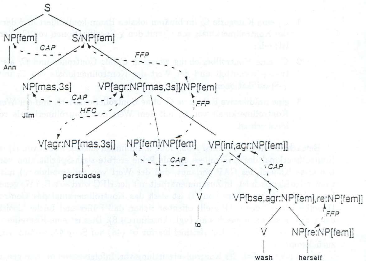
Abbildung 7: CAP und das Zusammenwirken der MIPs
