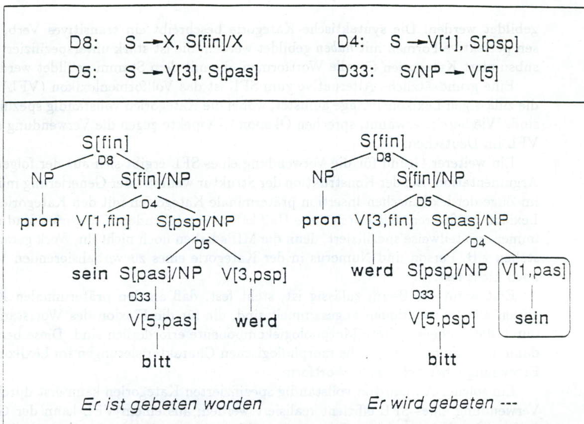
Abbildung 19: Zur lexikalischen Beschränkung syntaktischer Strukturen
