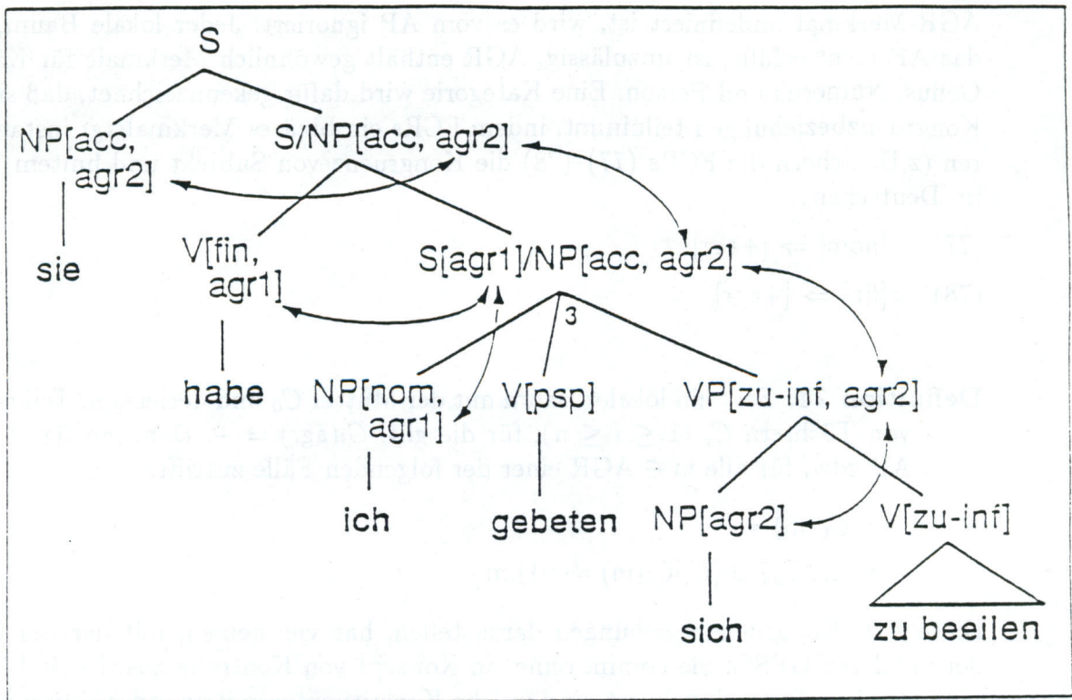
Abbildung 11: Kongruenzbeziehungen mit dem revidierten AP
