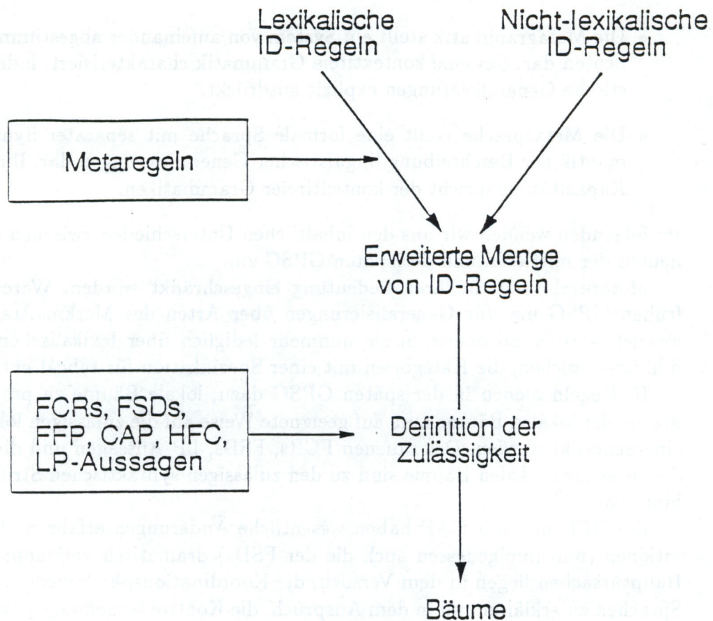
Abbildung 3: Die Organisation der späten GPSG
