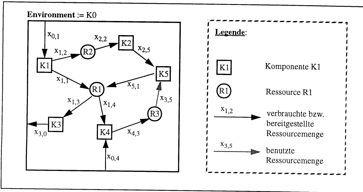
Bild 3.1: Graphische Veranschaulichung einer ressourcen-orientierten Modellierung
