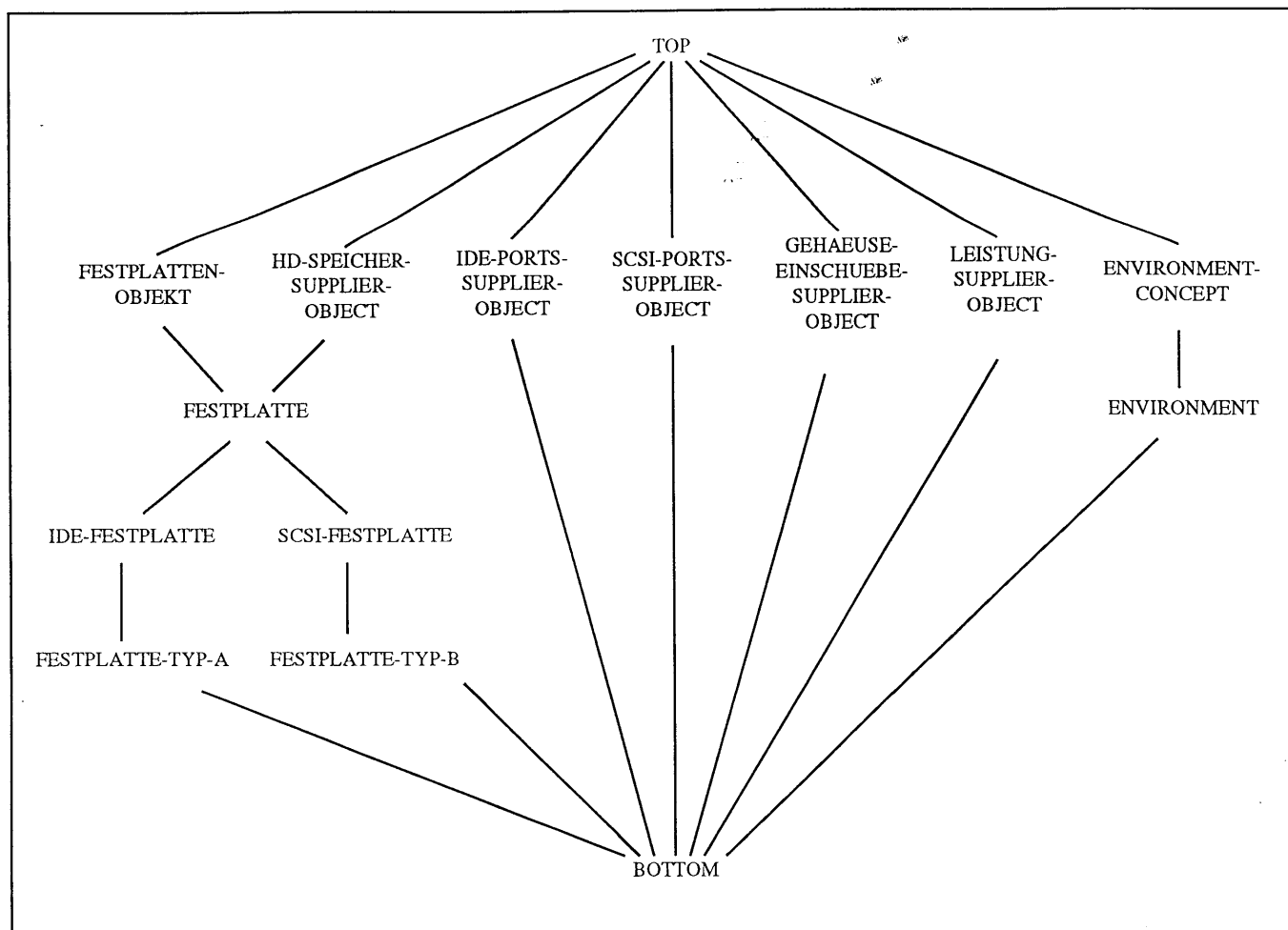
Bild 6.1: Graphische Darstellung der Taxonomie
