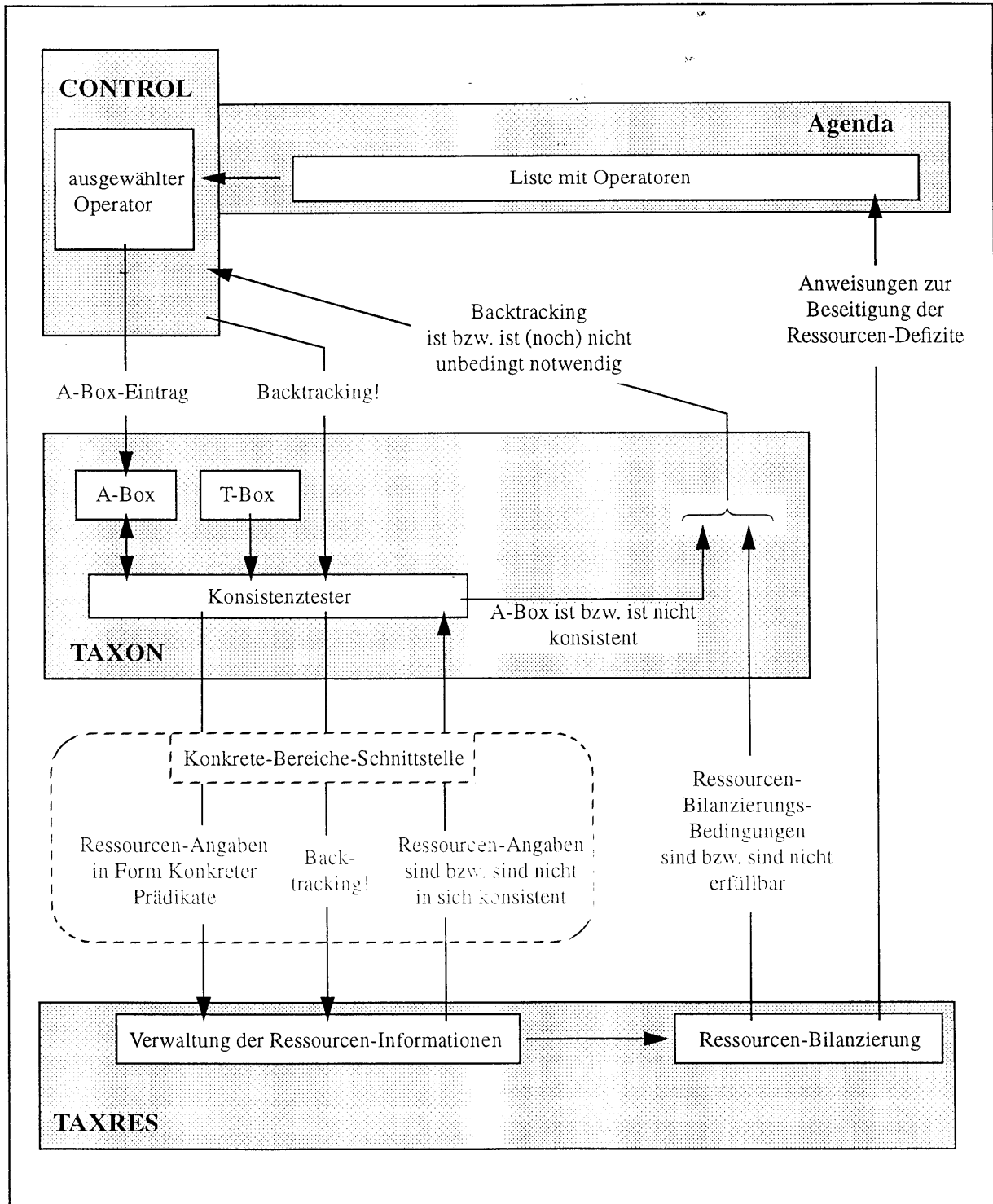
Bild 4.3: Der Informationsfluß zwischen TAXRES, TAXON und CONTROL
