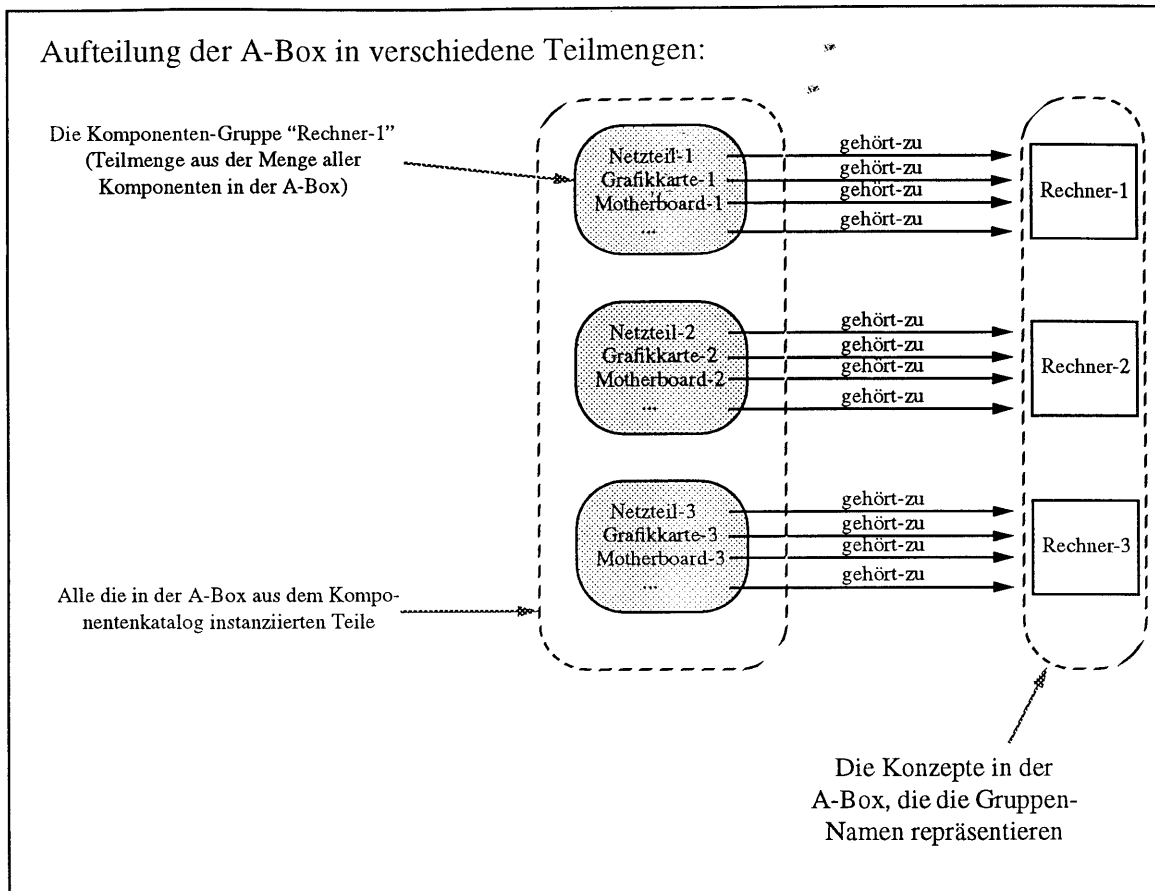
Bild 7.1: Graphische Veranschaulichung lokaler Ressourcen
