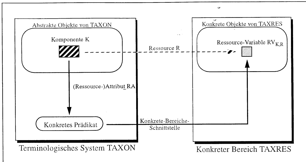
Bild 5.1: Veranschaulichung, wie einer Komponente aus TAXON indirekt über Konkrete Prädikate eine Ressource-Menge aus TAXRES zugewiesen wird
