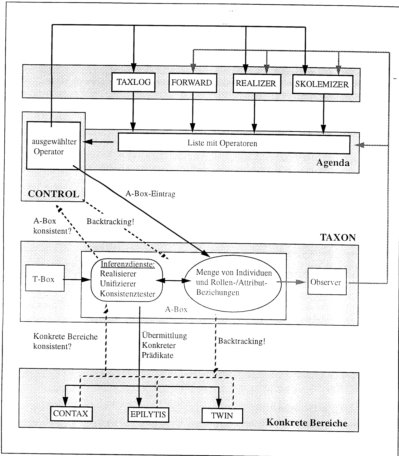
Bild 2.1: Die Architektur und der Informationsfluß im TOOCON-Werkzeugkasten
