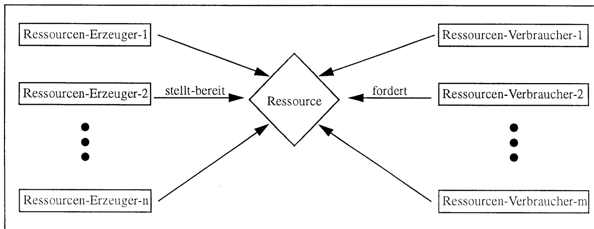
Bild 3.2: Die n:m-Beziehung zwischen Komponenten, die Ressourcen bereitstellen und Komponenten, die Ressourcen benötigen
