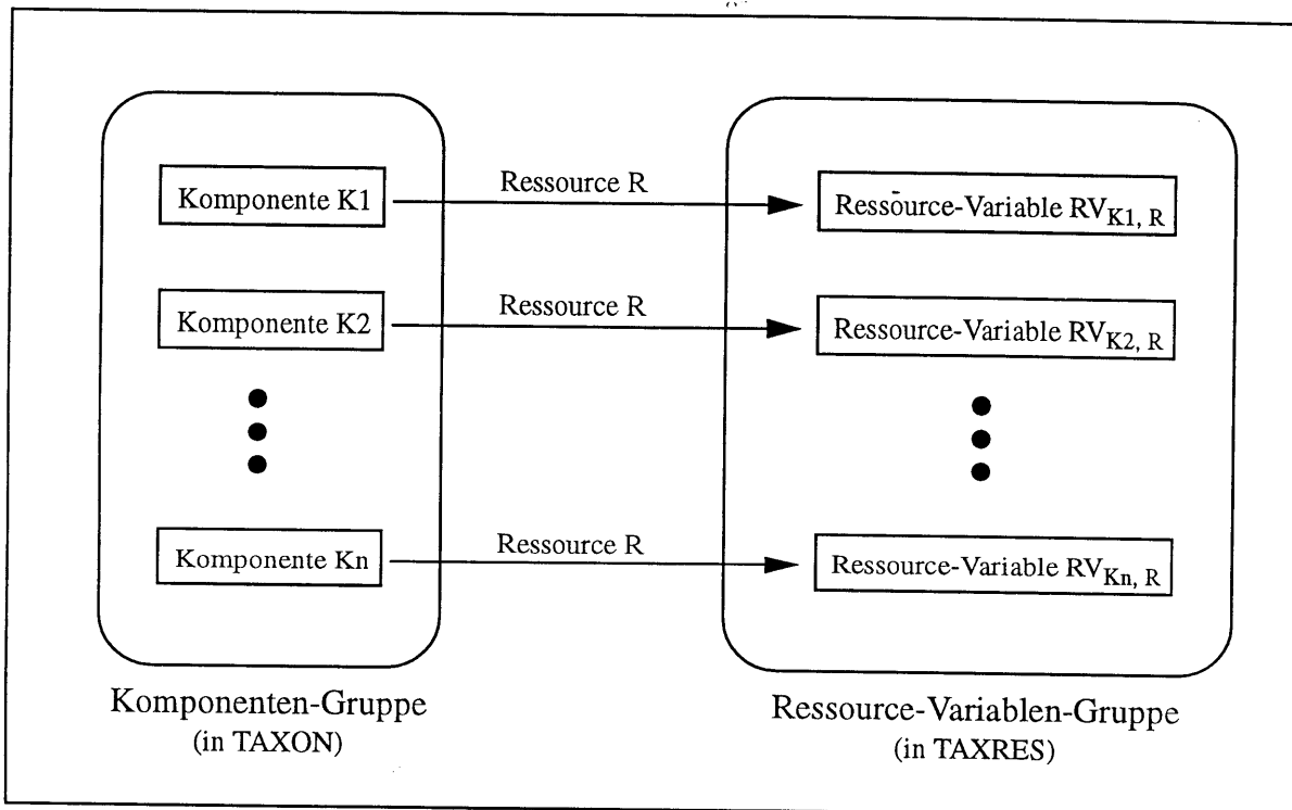
Bild 7.2: Die Repräsentation einer lokalen Ressourcen-Bilanzierungs-Gruppe
