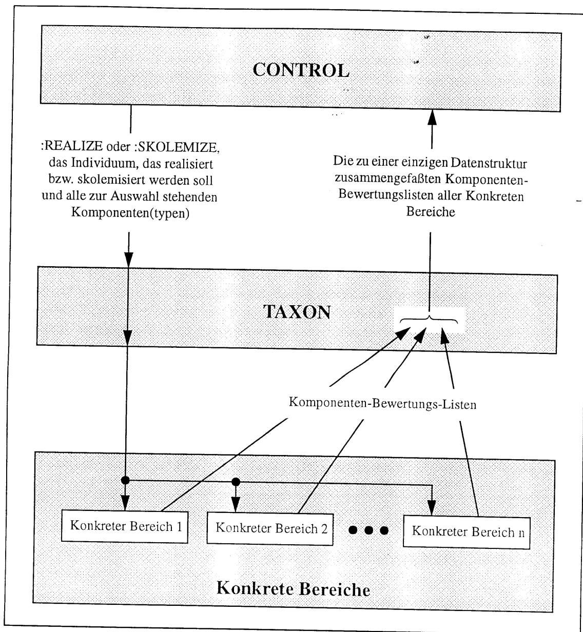
Bild 5.2: Die Schnittstellen-Erweiterungen um CONTROL bei der Komponenten-Auswahl zu unterstützen
