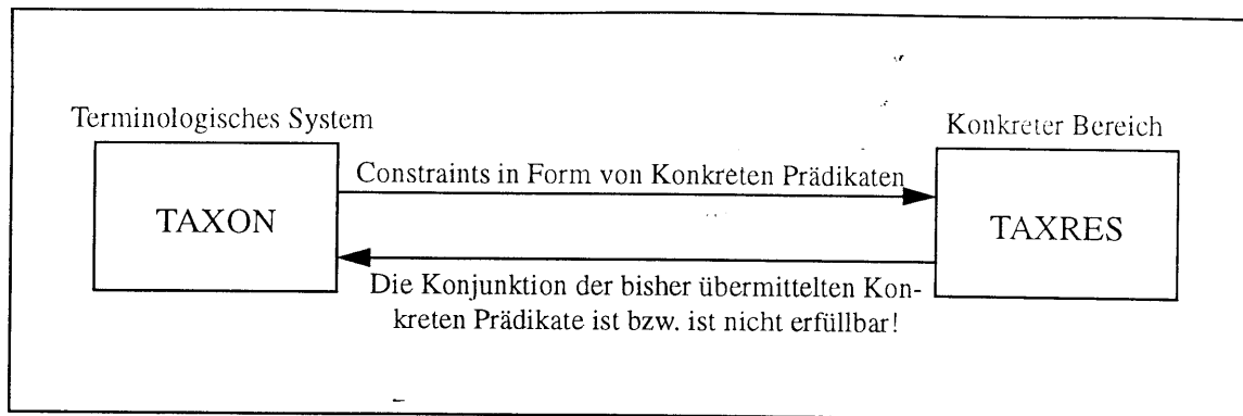
Bild 4.1: Die Konkrete-Bereiche-Schnittstelle zwischen TAXON und TAXRES
